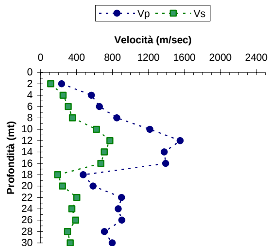
VELOCITA' SISMICHE
