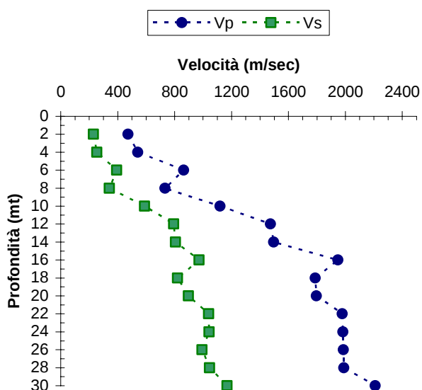
VELOCITA' SISMICHE
